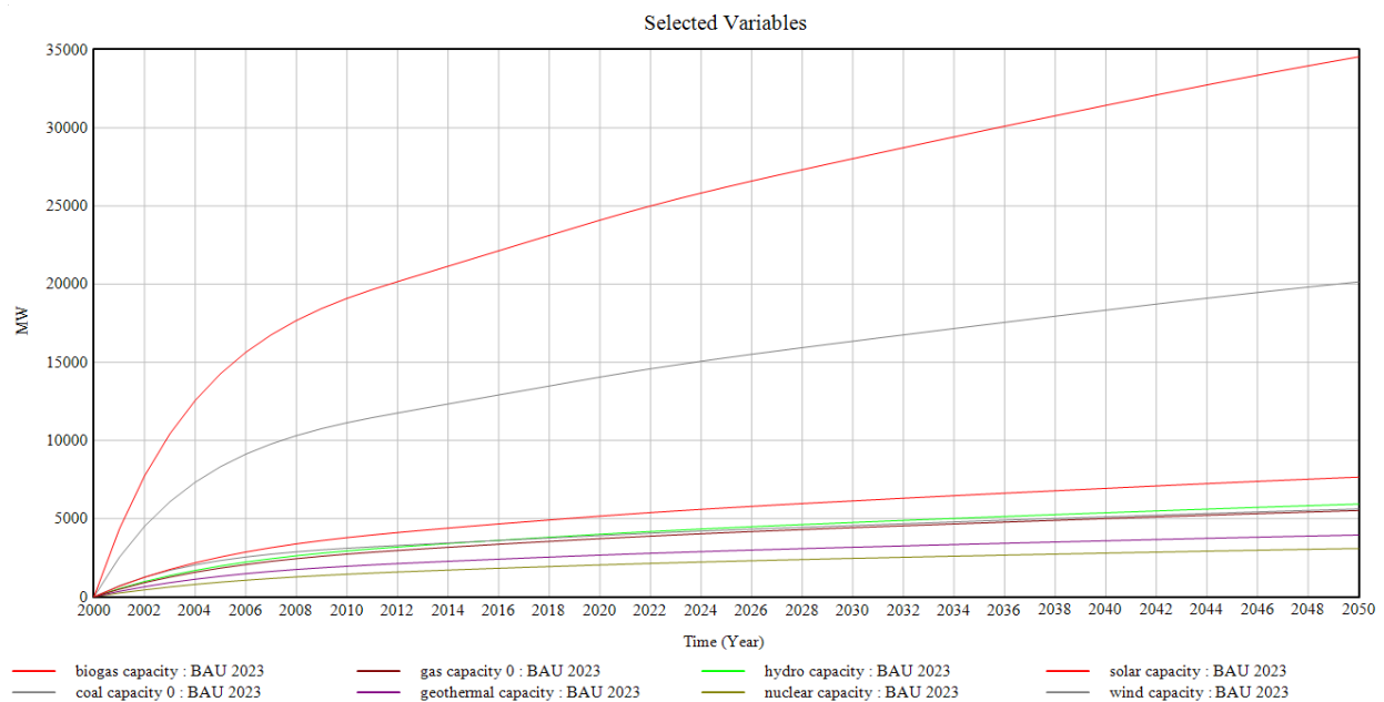
Рисунок 1 Необходимая установленная мощность для обеспечения спроса на электроэнергию при использовании одного из источников генерации, МВт
